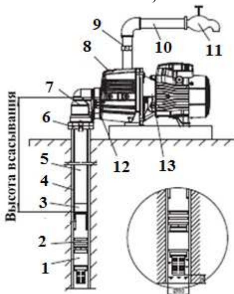
Рис. 3. Схема установки насосов моделей AJDm55/2H, AJDm75/2H, AJDm110/2H.
