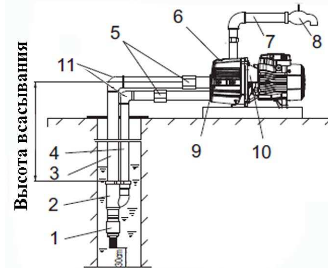
Рис. 7. Схема установки насосов моделей AJDm55/4H, AJDm75/4H, AJDm110/4H.
